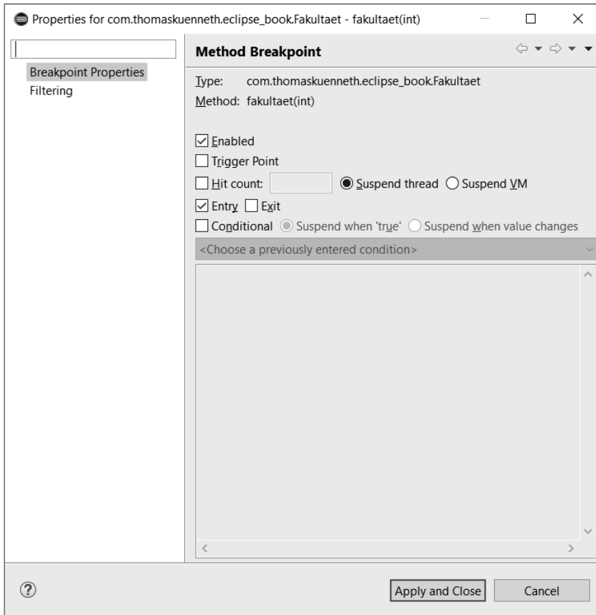
Bild 4.16 Eigenschaften eines Method Breakpoints
