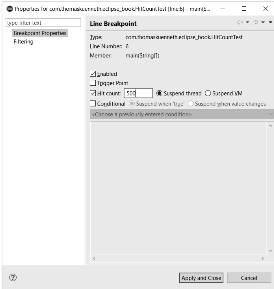
Bild 4.22 Festlegen eines Hit Counts
