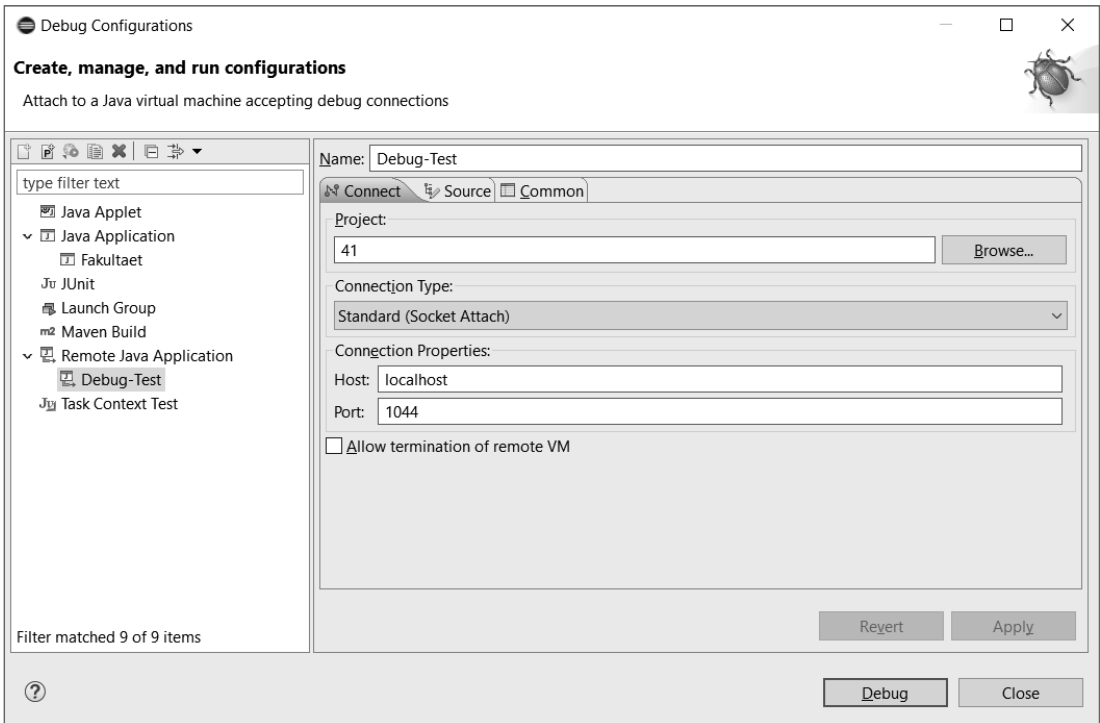
Bild 4.12 Anlegen einer neuen Remote Launch Configuration
