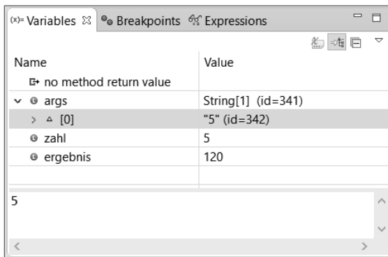
Bild 4.10 Die Sicht „Variables“
