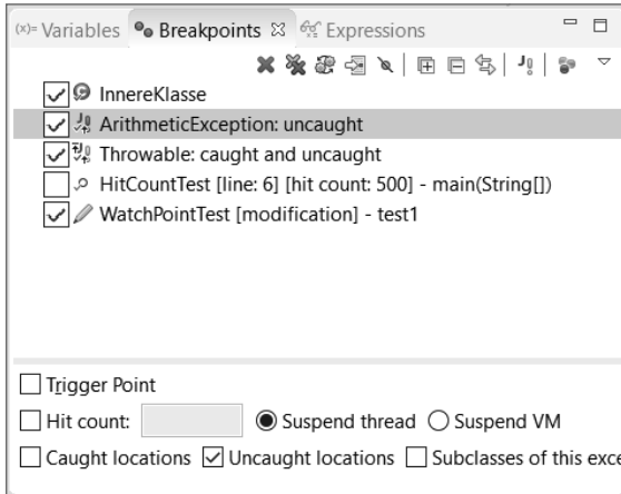
Bild 4.23 Breakpoint mit Hit Count nach dem ersten Halt
