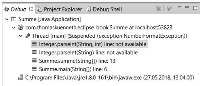
Bild 4.29 Stack Trace nach der Ausnahme „NumberFormatException“
