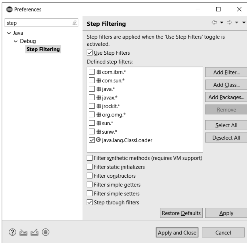
Bild 4.25 Die Seite „Step Filtering“ des Dialogs „Preferences“
