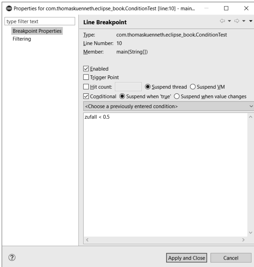
Bild 4.24 Eigenschaften eines bedingten Breakpoints
