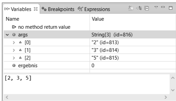
Bild 4.28 Die Sicht „Variables“ nach Ändern der Variablen „args“
