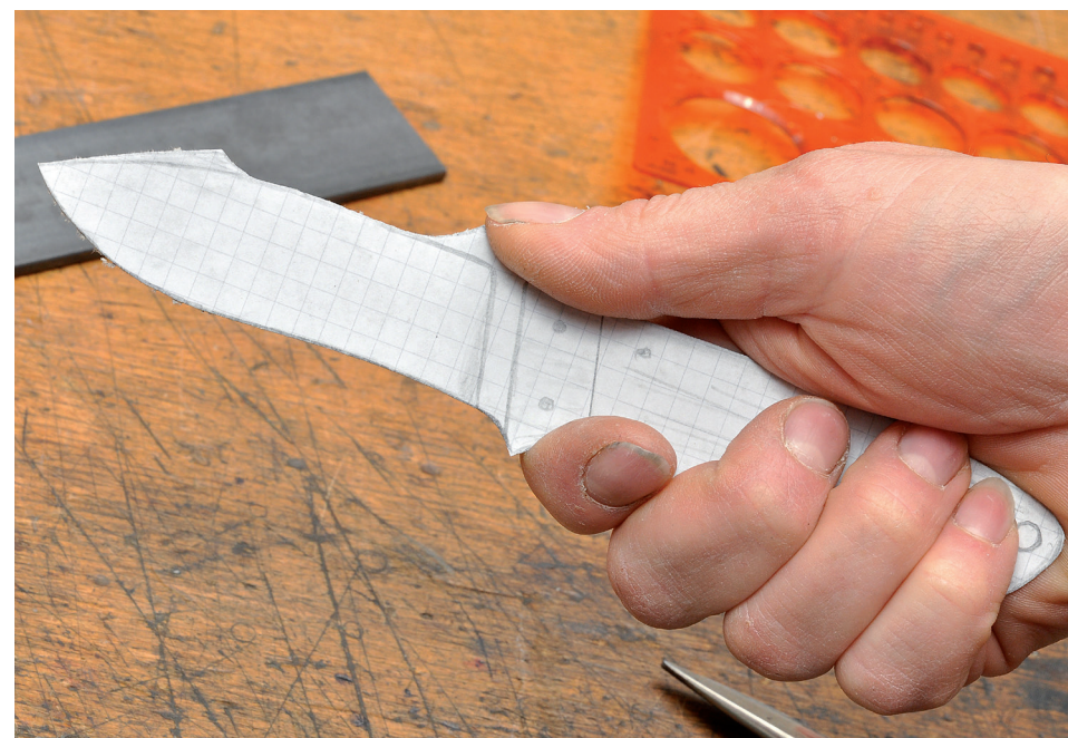
Prüfung der Handlage: Haben die Finger Platz, sind die Fingermulden angenehm, sitzt die Daumenauflage an der richtigen Stelle?
