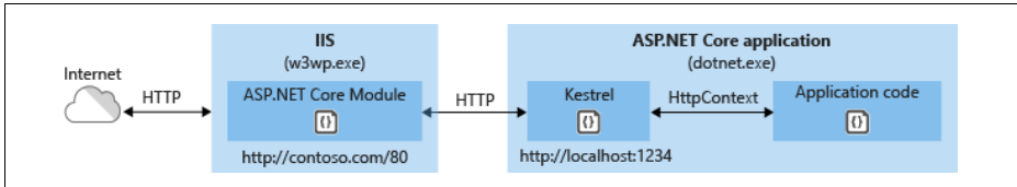
Abbildung 9-34: Integration von Kestrel in die IIS (Urheber: Microsoft ( docs.microsoft.com/en-us/aspnet/core/fundamentals/servers/aspnet-core-module ))
